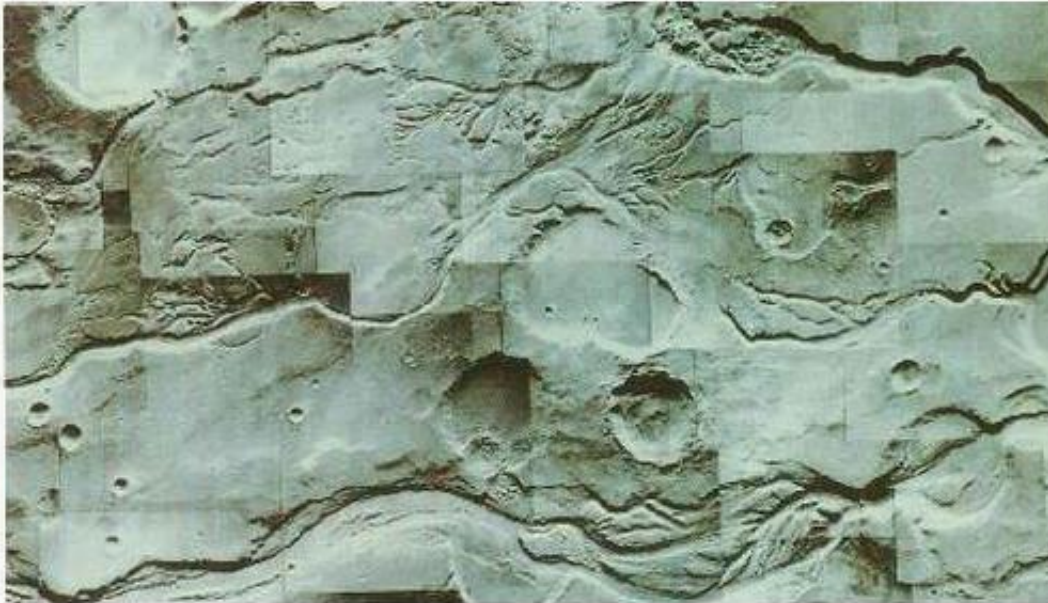
Mars Dry Rivers
